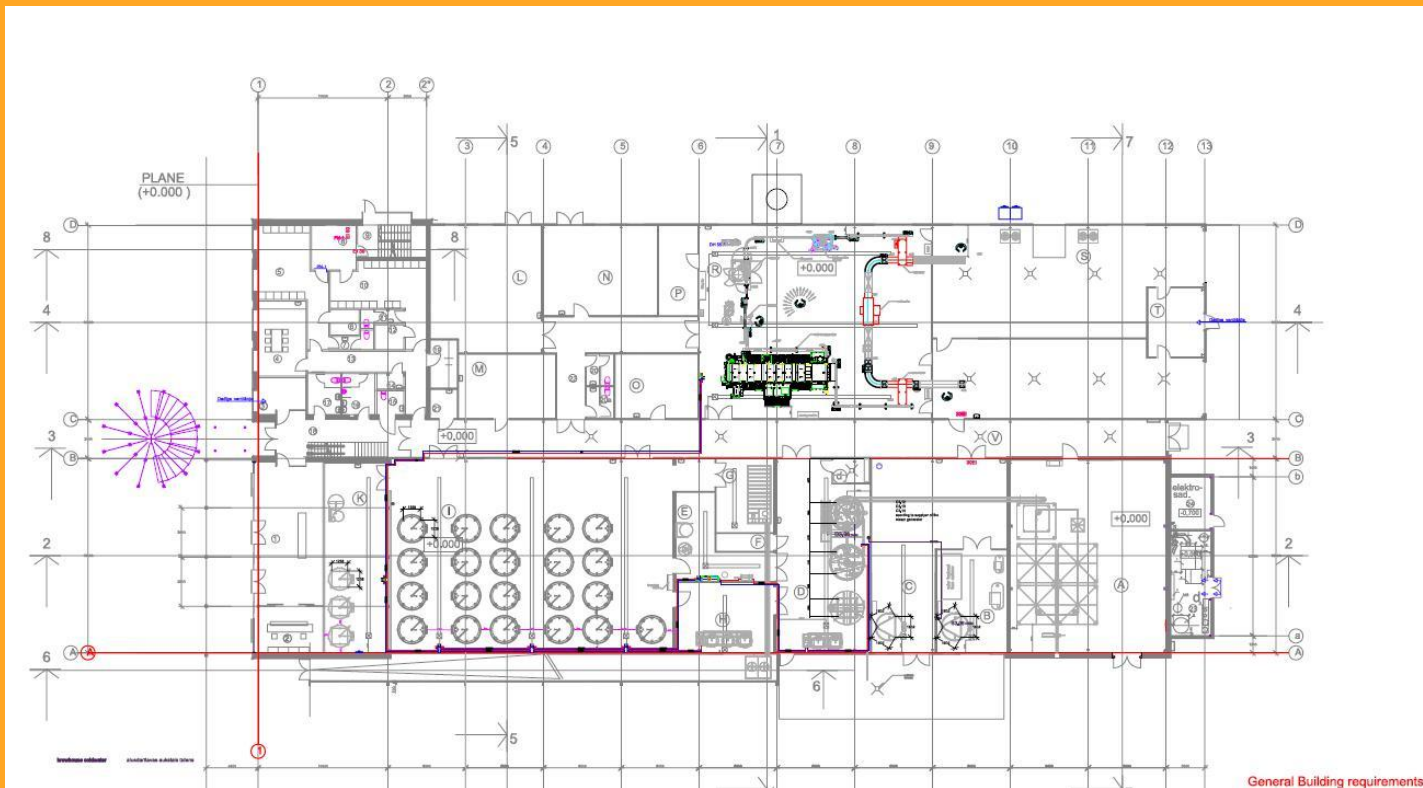
Промышленная пивоварня 6000 л за одну варку
